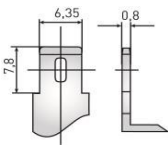
Клеммы нож F2
