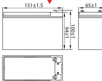
РАЗМЕРЫ
