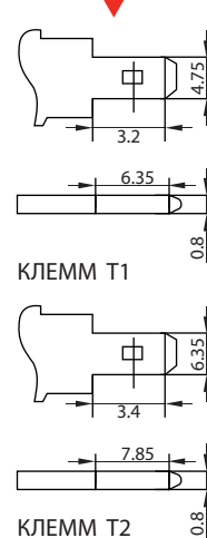
ТИП КЛЕММ
